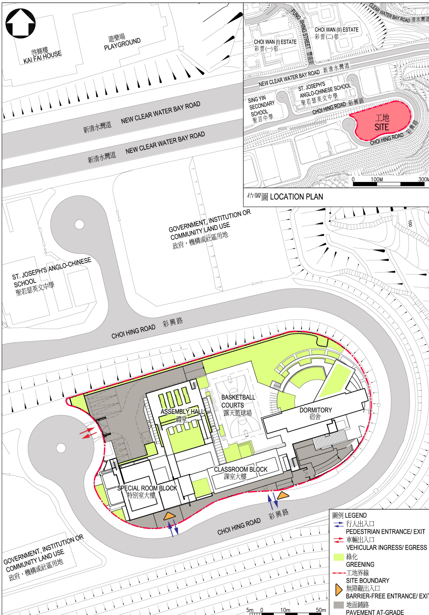
工地平面圖 SITE PLAN
