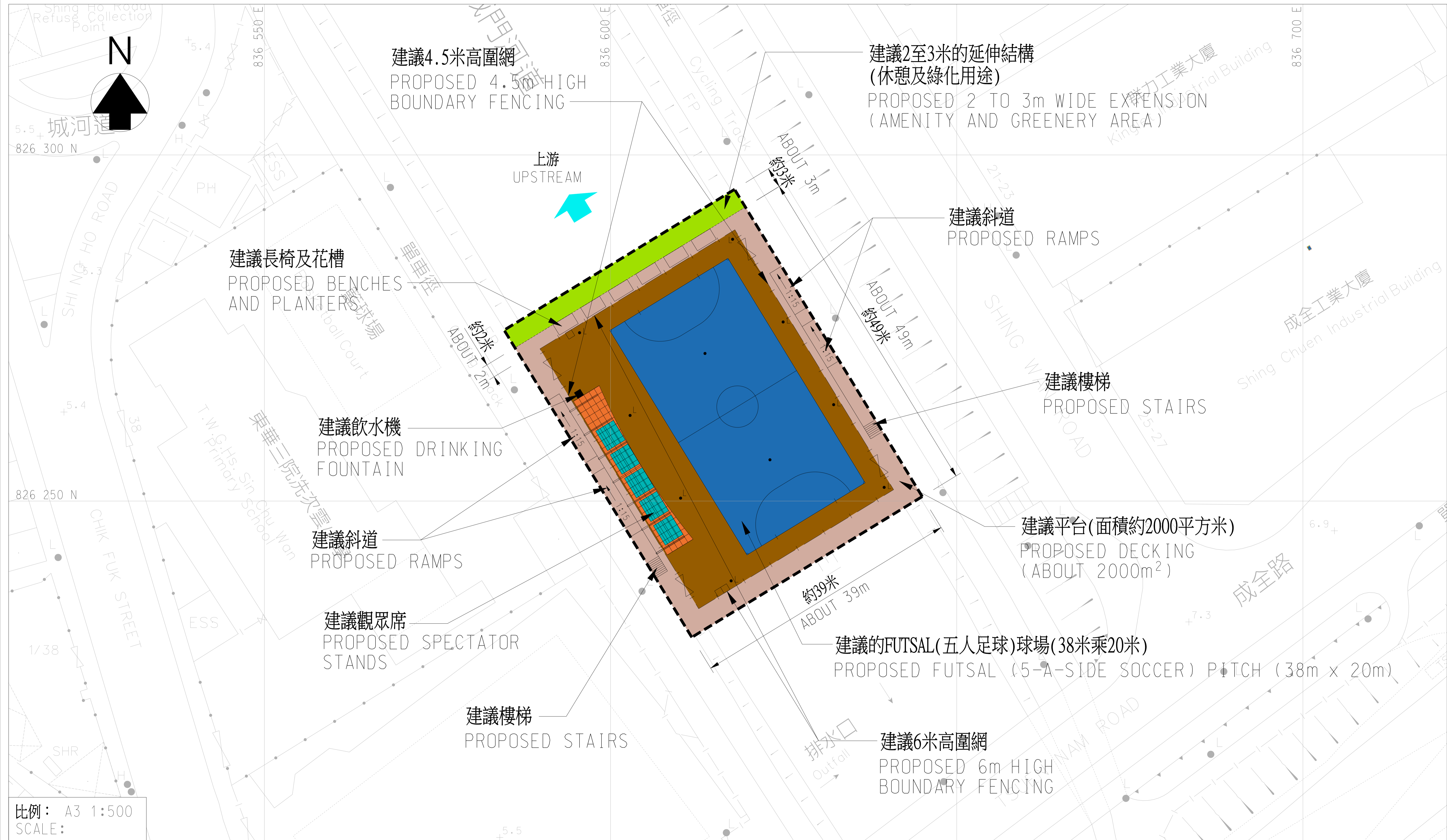
覆蓋沙田大圍明渠- 平面佈局圖
