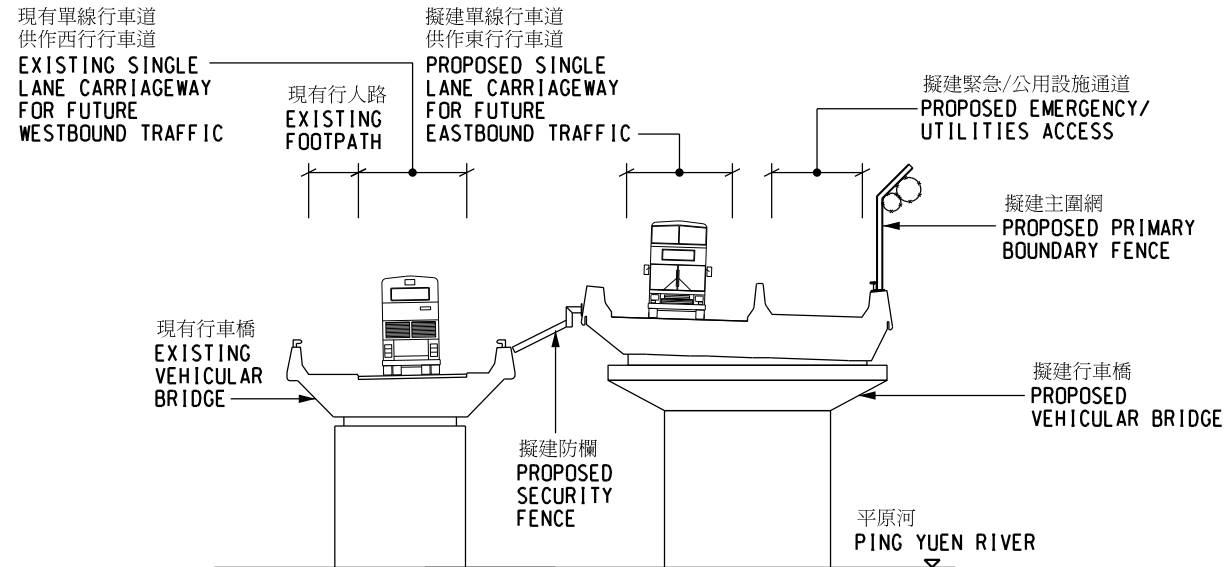
橫切面 SECTION 1-1
