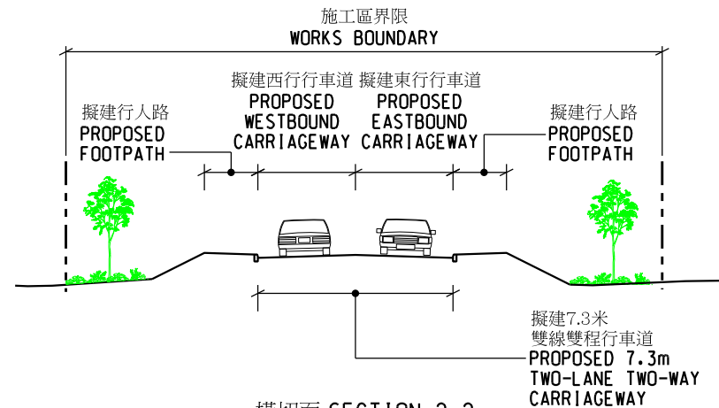
橫切面 SECTION 2-2
